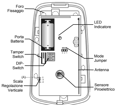
Figura B.1: Sensore PIR senza copertura MS845
