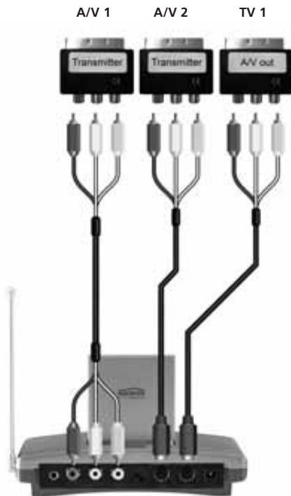
Abbildung 1 A/V SENDER
