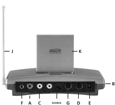
Afbeelding 3 A/V ZENDER
