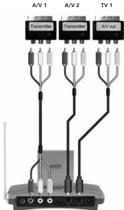
Image 1 EMETTEUR A/V
