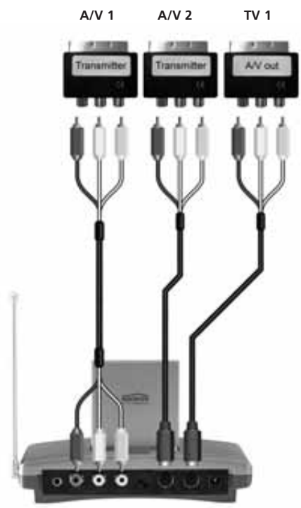
Figura 1 EMISOR A/V
