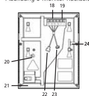
Abbildung 5 Monitor Rückseite
